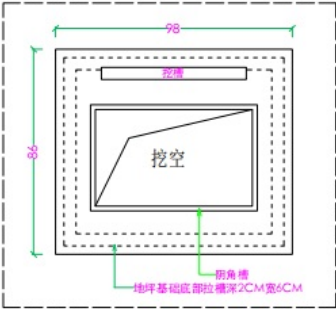
地坪加工示意
