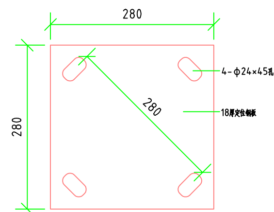
定位钢板大样图
