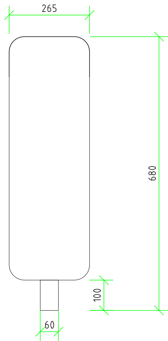
7米高路灯灯头俯视图
