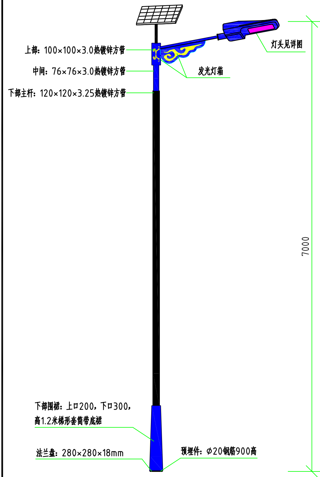
7米高路灯大样图
