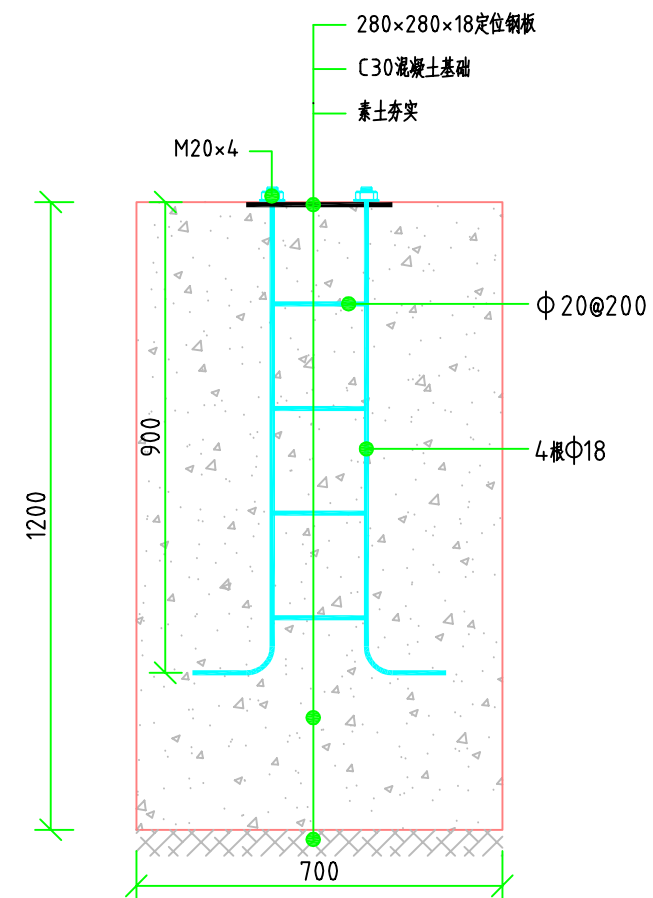
路灯基础剖面图
