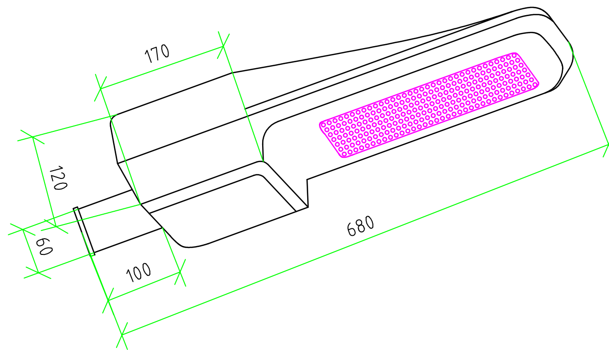
7米高路灯灯头立体图
