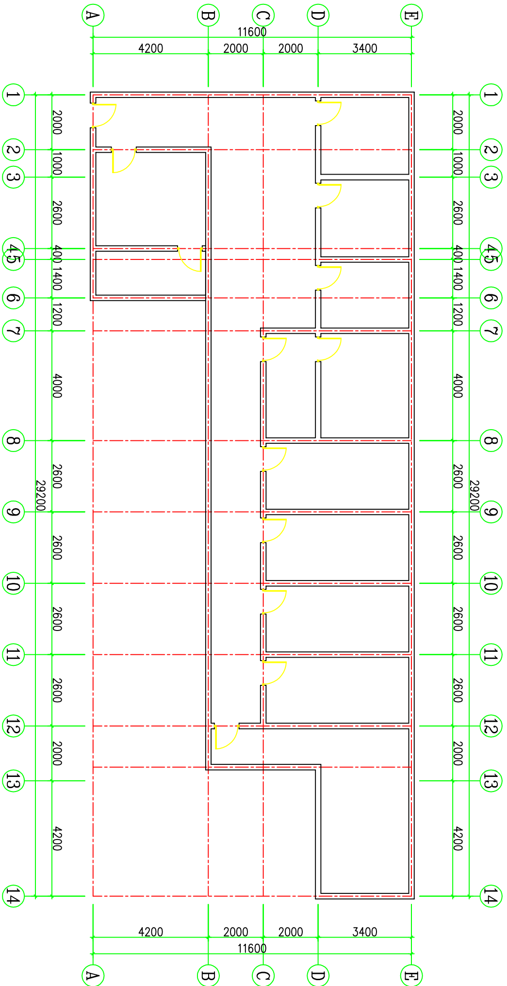
敖镇派出所执法办案中心平面图
