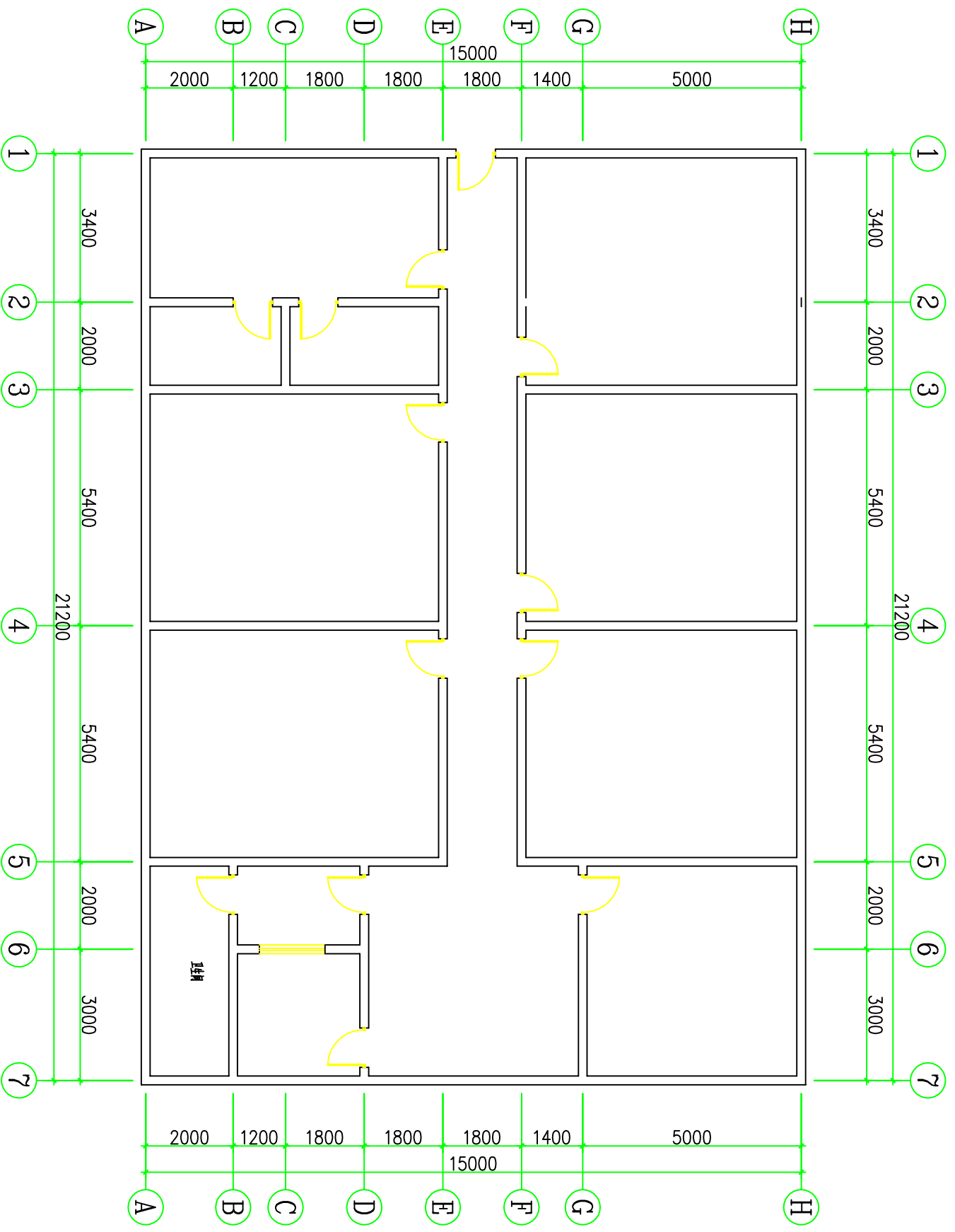
上海庙派出所执法办案中心平面图
