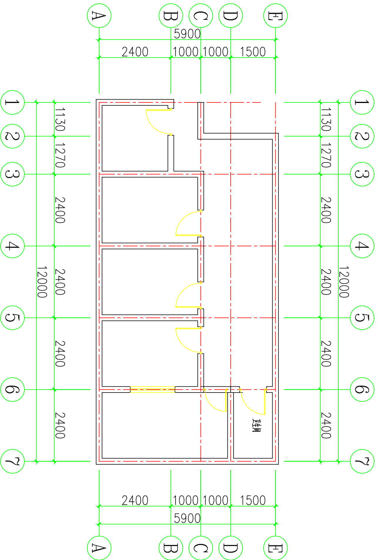
城川派出所执法办案中心平面图
