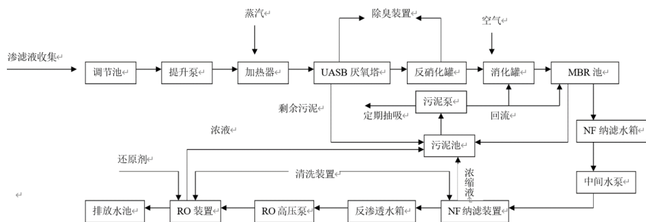
项目工艺流程图
