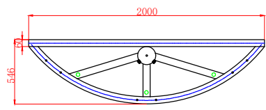
灯盘示意图
