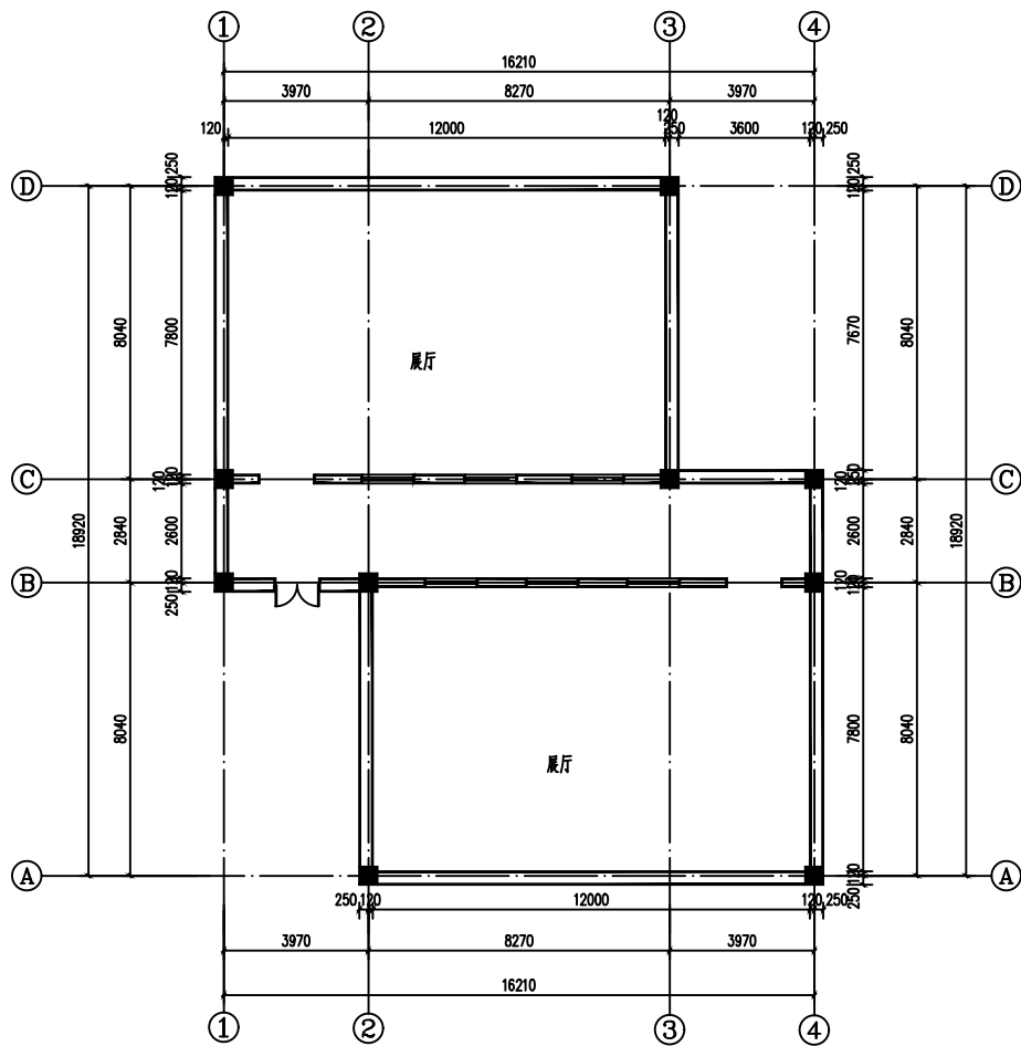
西1平面示意图 1:100
