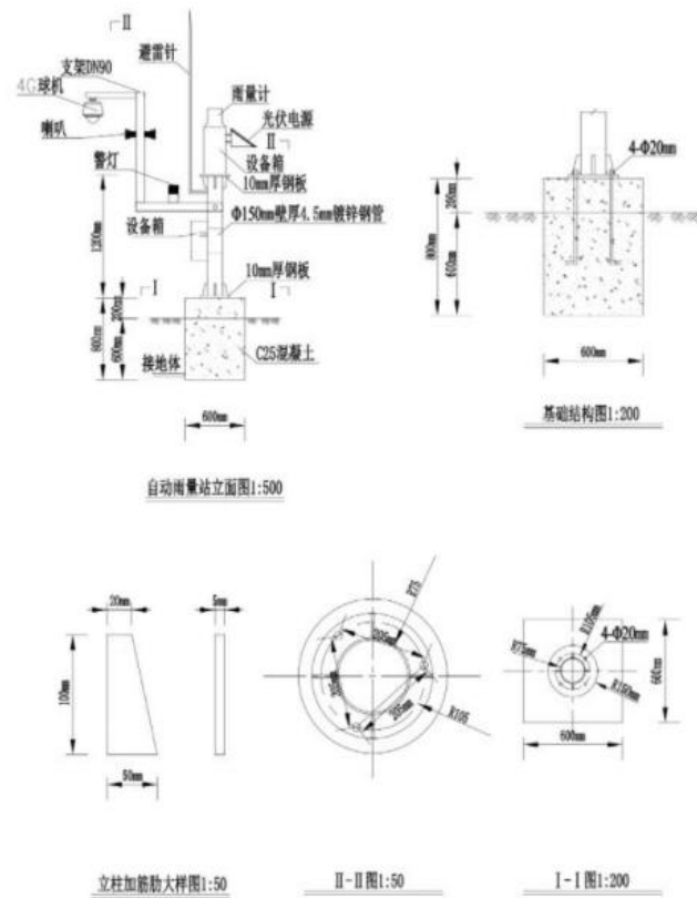
图 3-6-1 雨量站安装结构示意图
