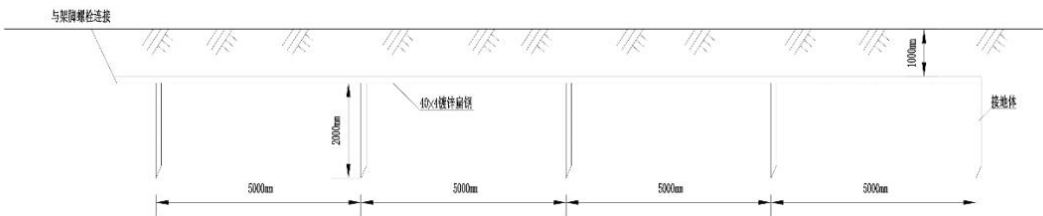
图 1-7 避雷针图
