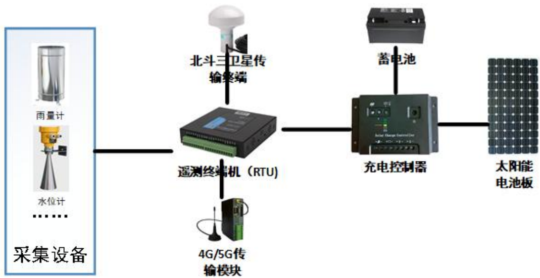
图 1-3 主要设备组成结构图
